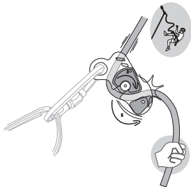
Fig.2 Function principle / Principe de fonctionn
